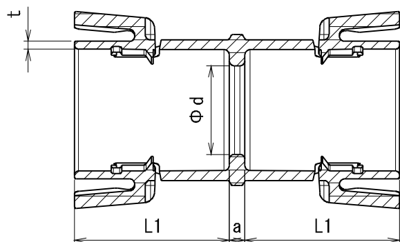
断面 A-A
